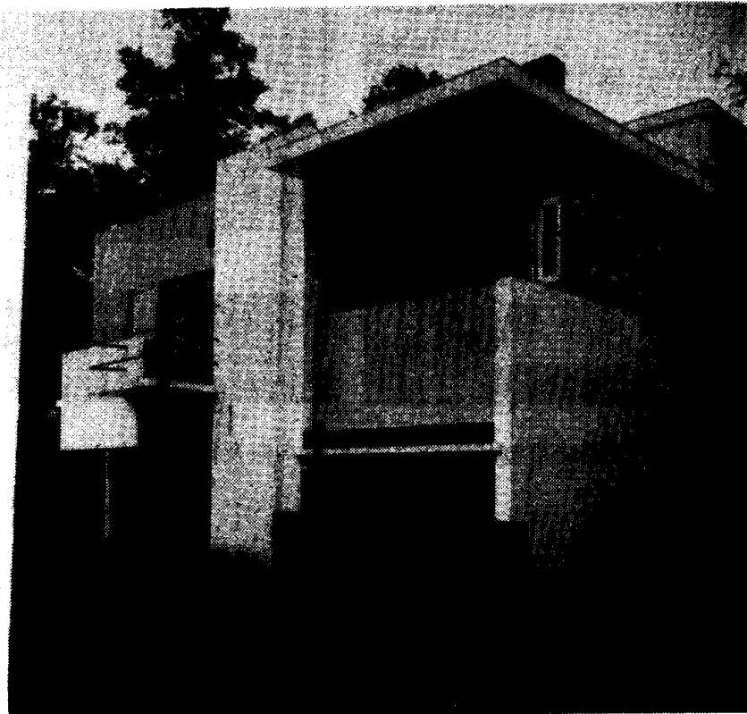
图 14 荷兰乌德勒支市施罗德住宅，里特维德，1924 年
