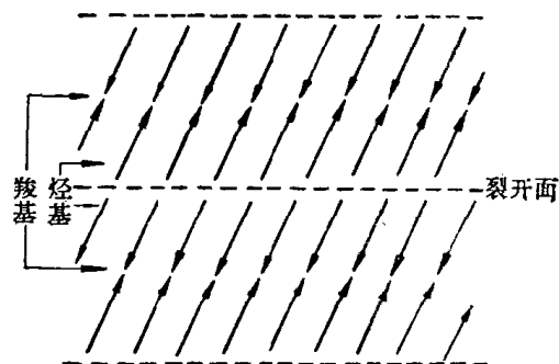
图 12-1 羧酸结晶中碳链的排列
