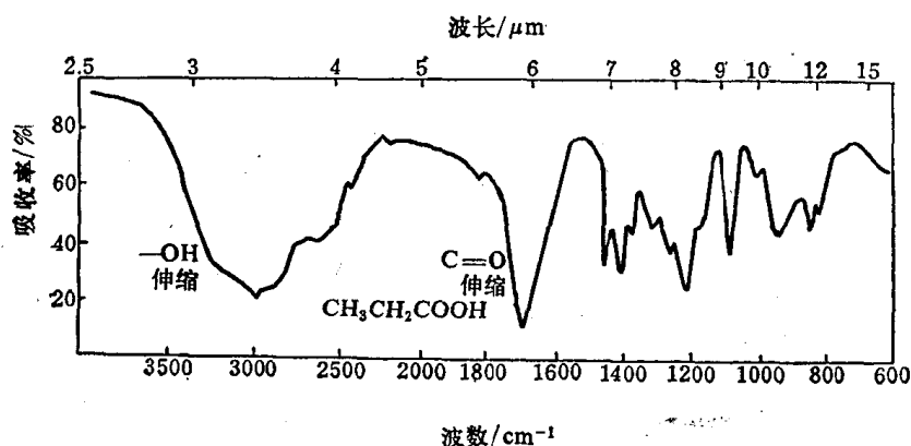
图 12-2 丙酸的 IR 图
