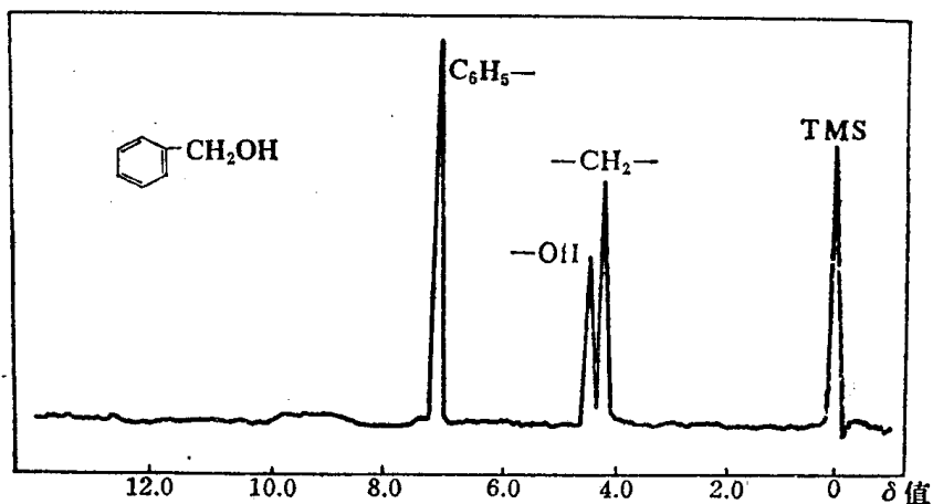
图 12-4 苧醇在 CCl 4 中的 NMR 图
