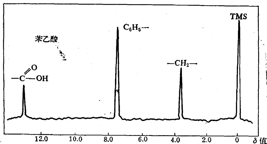
图 12-3 苯乙酸在 CCl_4 中的 NMR 图
