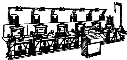
560—6—10型连续拉丝机 进线 \phi 6.5 mm 出线 \phi 2 mm
