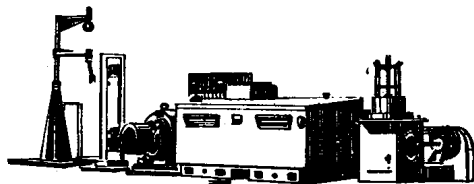
LT—11/450 水箱拉丝机 最大进线 高碳钢 \phi 4 m/m 铜材 \phi 8 m/m 最小出线 \phi 1.5 m/m
