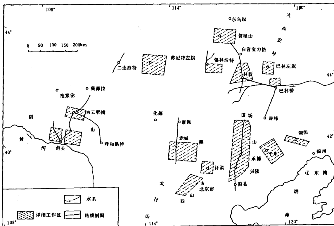
图 1-2 工作区路线图
