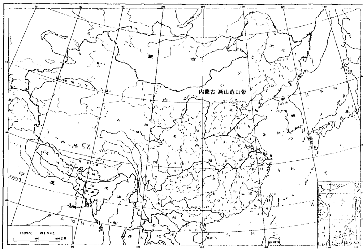
图 1-1 内蒙古-燕山造山带位置图
