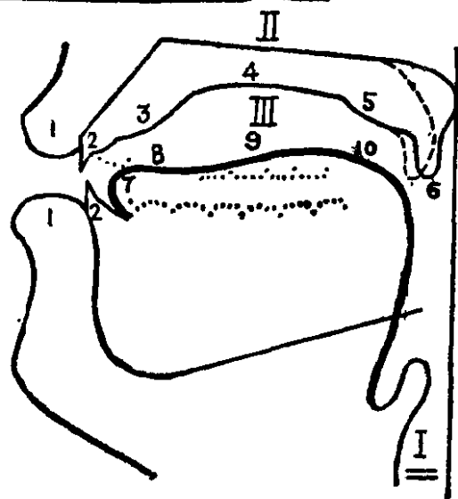
发音器官图
