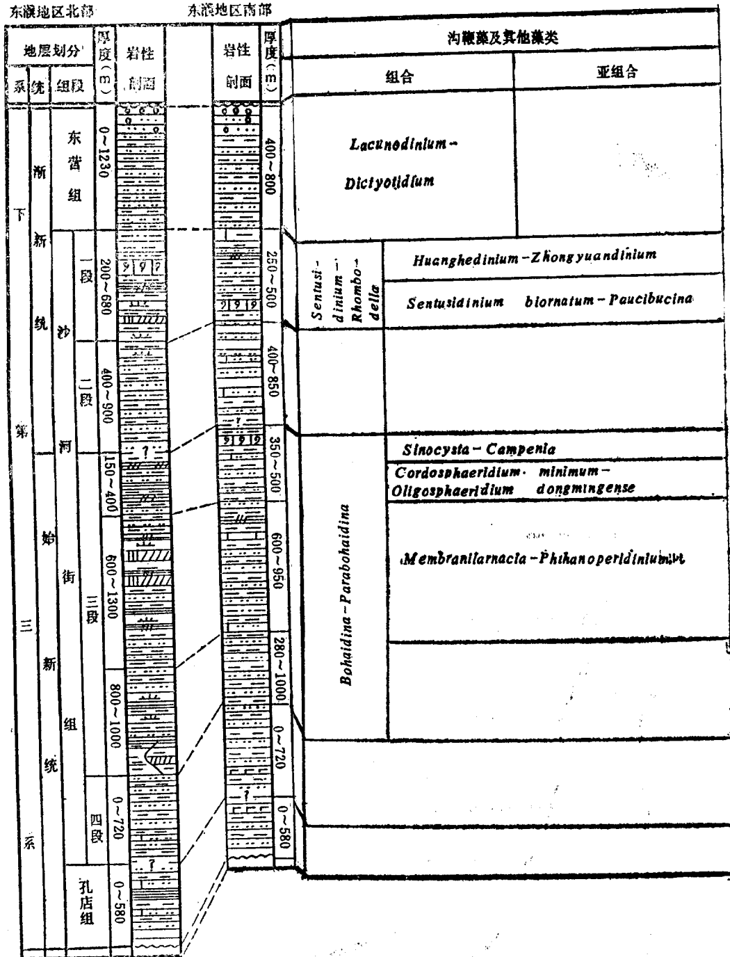
图2 东濮地区早第三纪沟鞭藻和其他藻类化石组合及地层柱状图
