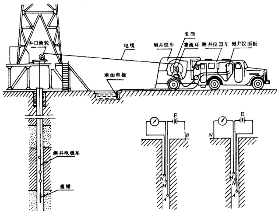
图 1.1 测井现场及电测井原理示意图
