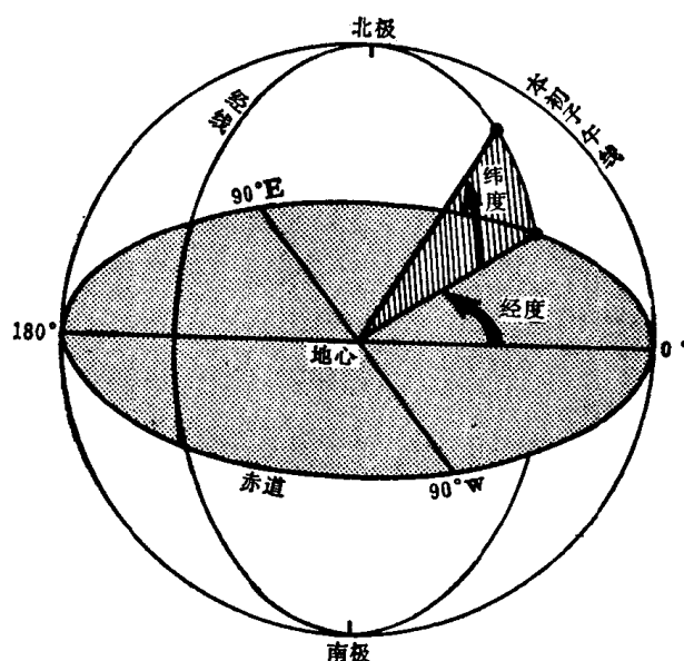
图 1.3 地理坐标: 纬度和经度
