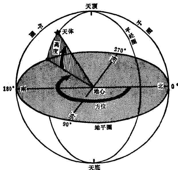
图1.5 天球地平坐标：高度和方位[角]
