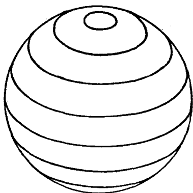
图1.1 纬 线
