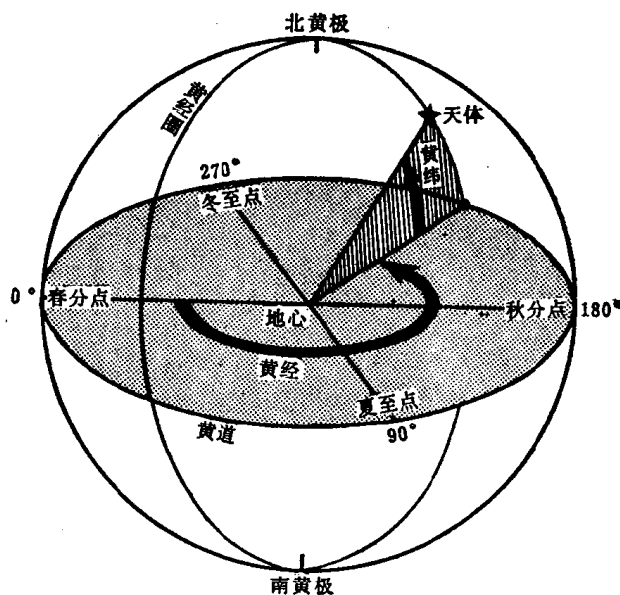
图 1.8 天球黄道座标:黄纬和黄经
