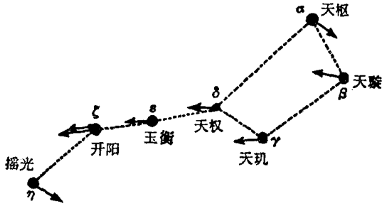
图 1.9 北斗七星的自行
