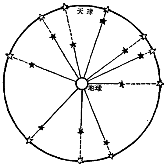
图1.4 天球示意图
