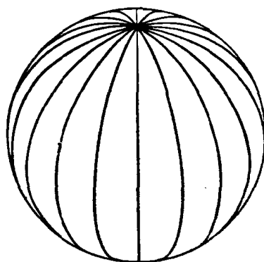
图1.2 经 线
