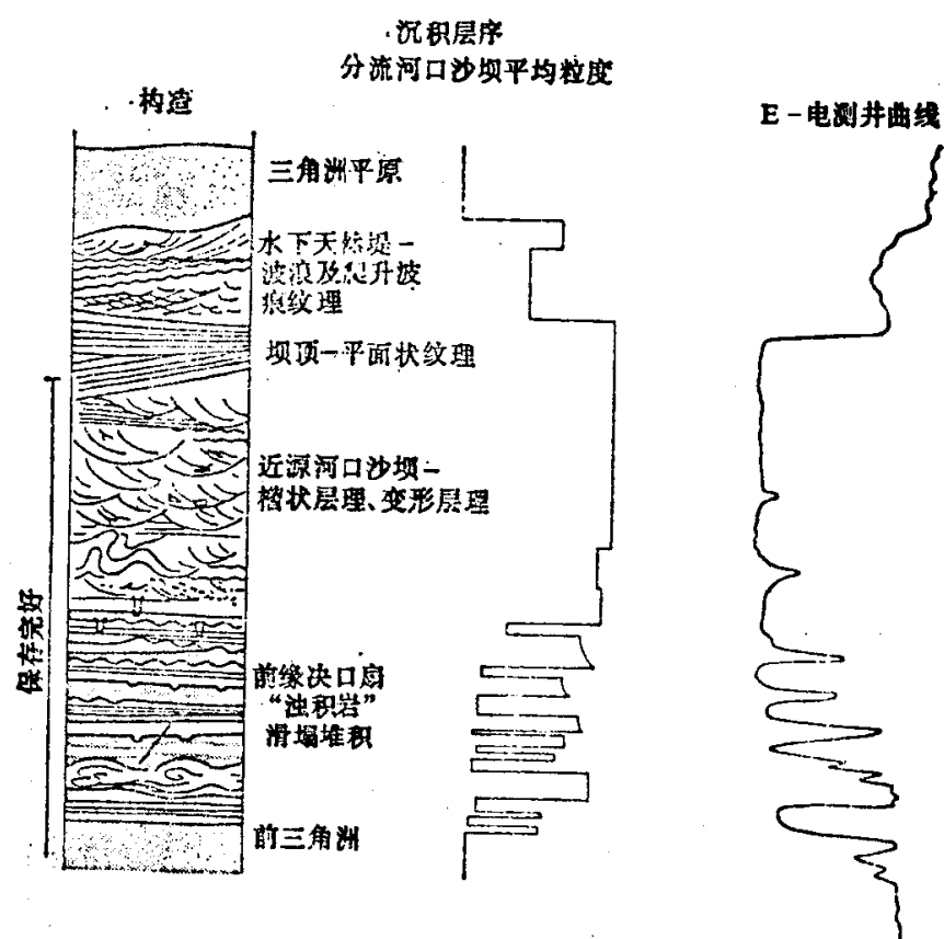
图 1-8 河口沙坝砂体综合垂直剖面 (据 Galloway 和 Hobday, 1983)
