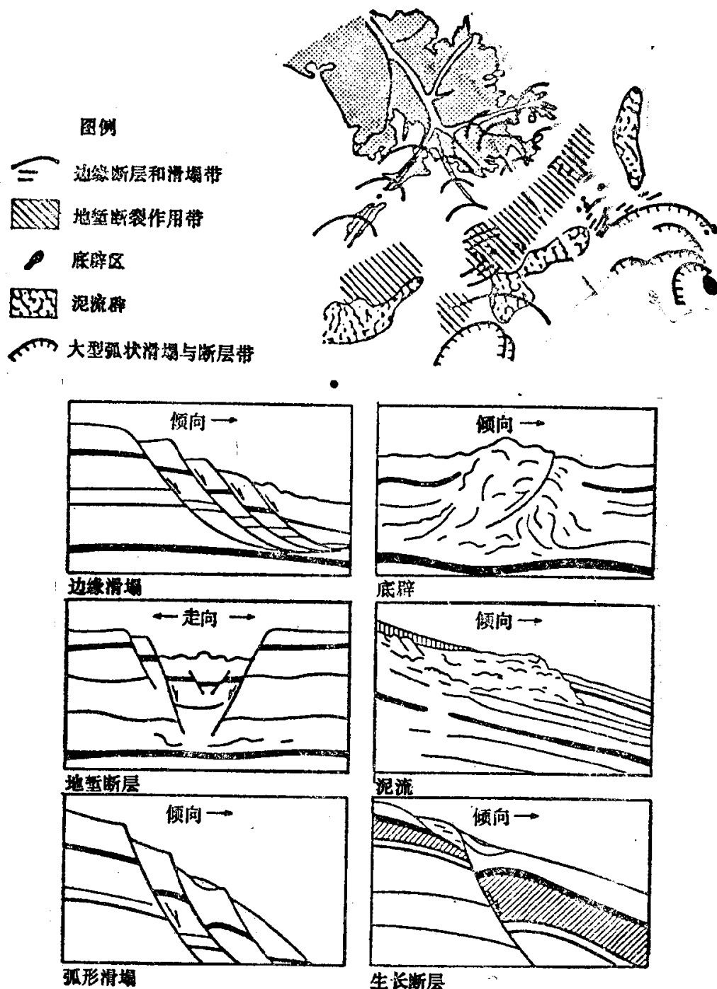
图 1-4 沿活跃进积的三角洲前缘发生的重力再沉积和变形作用型式 (据 Galloway 和 Hobday, 1983, 按 Coleman 和 Garrison 修改, 1977)
