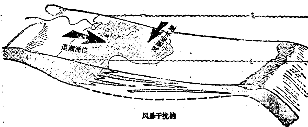
图1-10 受风暴干扰的陆架体系中砂的分布
