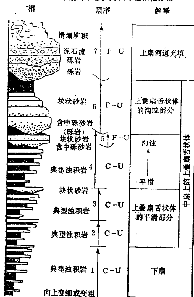
图 1-16 根据富砂扇状体的退覆建立的综合层序 (据 Walker, 1978)
