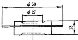
ZP200 型(配 SF12 散热器)
