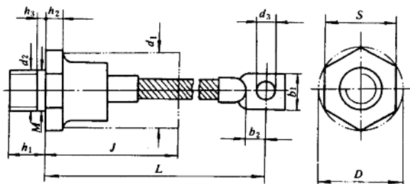
b) ZL081、12、16A、20A、24A
