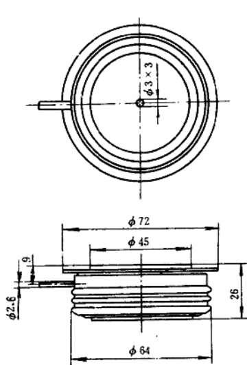
ZP500 型(配 SF-15 散热器)
