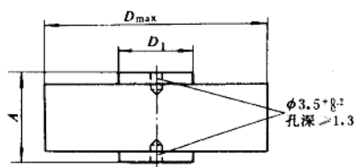
凸台形
