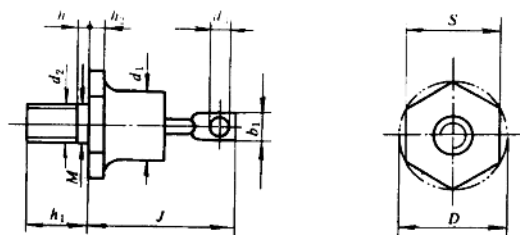
a) ZL05、06、08
