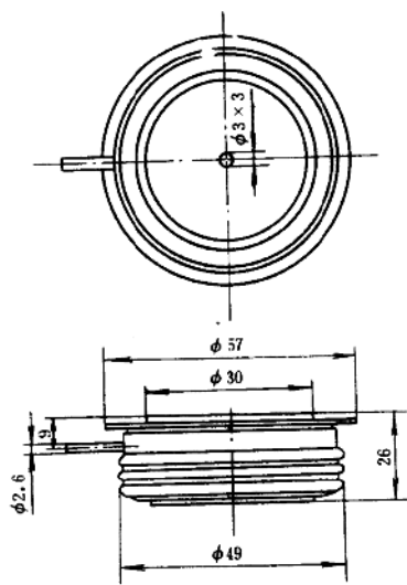
ZP200 型凹台(配厂标散热器)
