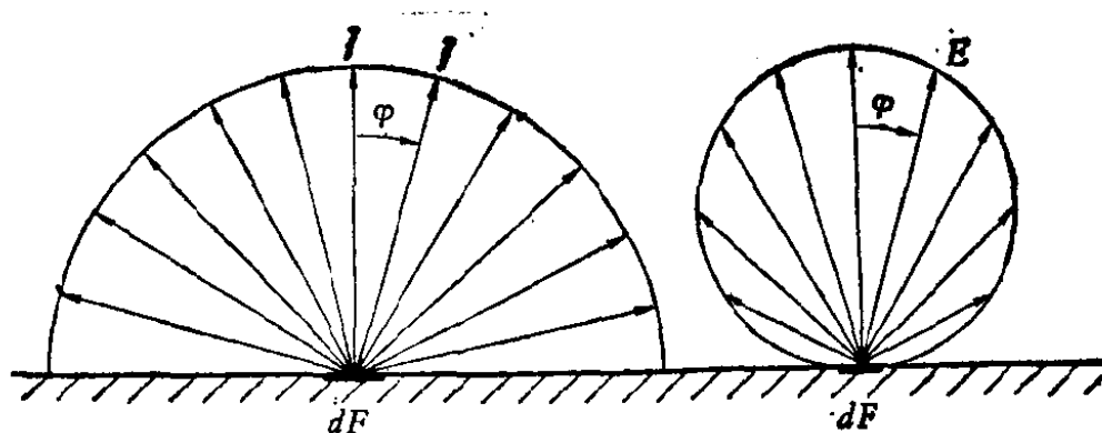
图 1-2 绝对黑体的辐射强度 J 和角辐射密度 E 的空间分布图
