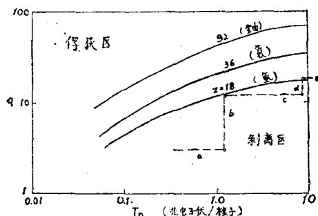
图2 密剥离器的计算离子平衡电荷态与能量的关系，其中 Z=18, 36 和 92 。虚线表示的是贝伐拉克中氙离子的加速过程和剥离，其中包括两次加速(a和c)，两次剥离(b和d)(见3.6节)。
