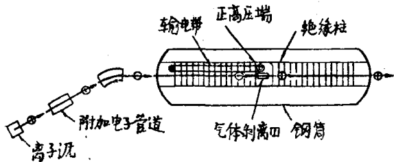
图7 串联静电加速器示意图〔取自范德格拉夫(18)〕。
