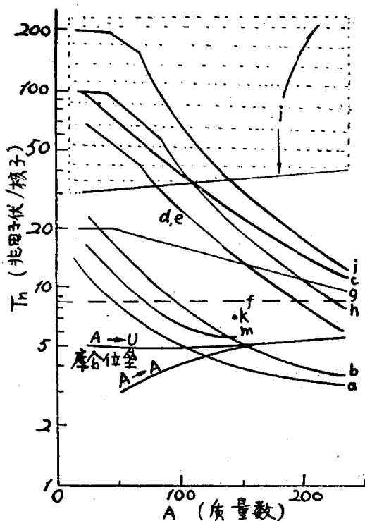
图6 几台加速器的单核能与质量数的关系。所用的符号在5节中说明。(a)HHIRF 串列静电加速器(T25); (b)HHIRF I阶段(T25+K90); (c)HHIRF II阶段(T25+K90+K400); (d) 巧克河(T13+K500); (e) 罗彻斯特(T13+K500); (f) 超级重离子直线加速器(D8.5); (g) UNILAC (D4.5+L23.8); (h) GANIL(K25+K400+K400); (i) MSU (K25+K500+K800); (j) 贝伐拉克(D8.5+S2.6) [仅给出了下限, 上限的单核能 T_n = 26 亿电子伏(对于 A = 20 ), 和 T_n = 13 亿电子伏(对于 A = 238 )]; (k) 杜布纳的JINR U200+U300; (m) JINR 的U400(K725)。
