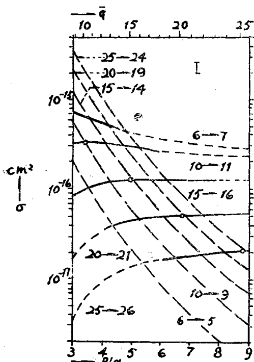
图1 空气中碘离子的电荷交换截面与离子速度的关系。速度用 \beta/\alpha 表示，其中 \alpha 是精细结构常数，等于 1/137 。图上面刻度是剥离离子平均电荷态 \bar{q} [取自参考文献(12)]。
