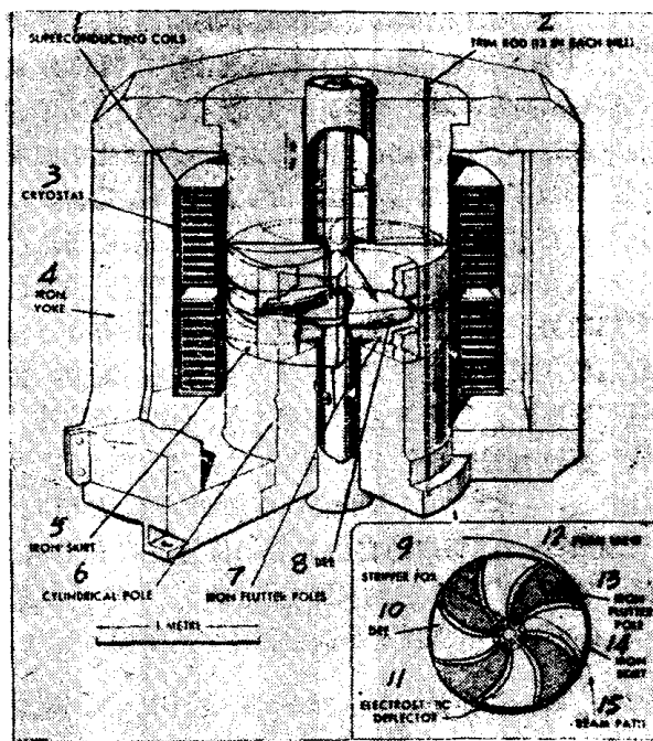
图19 加拿大巧克河建造中的超导回旋加速器。插图示出了外部注入方法。剥离膜放在中心区附近来降低粒子磁刚度, 使它在第一圈就被俘获。
