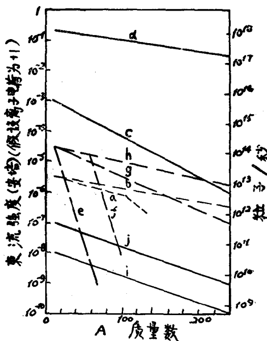
图5 重离子加速器的束流强度与质量数的关系。(a)25兆伏串联静电加速器; (b)串联静电加速器 + 回旋加速器; (c)现有的直线加速器; (d)用于重离子聚变反应的强流直线加速器; (e) K = 140 的现有回旋加速器; (f)计划中的 K = 500 的超导回旋加速器; (g)计划中的串联回旋加速器, 其中每个加速器的 K = 400 ; (h)计划中的串联超导回旋加速器, 其中一个 K = 500 , 另一个 K = 800 ; (i)直线加速器和同步加速器 (完成束流改进计划后的贝伐拉克); (j)直线加速器 + 同步加速器 (重复频率20赫)。
