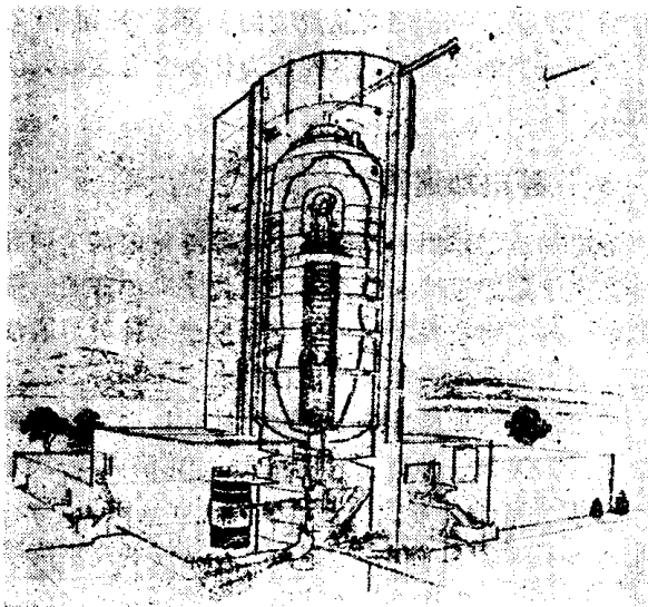
图8 由NEC造的HHIRF25兆伏串联静电加速器剖视图。从离子源出来的负电荷束流弯转90°，向上加速到端部，并在这里剥离，弯转180°后，再向下加速。90°磁铁可绕垂直轴转动，这样就可将束流送到任何一条径向输运线。
