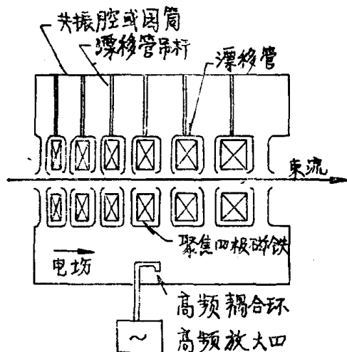
图10 漂移管高频直线加速器示意图
