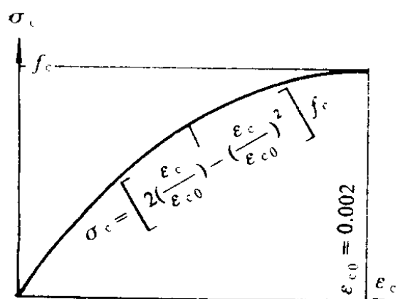
图 2-1 混凝土轴心受压 应力-应变关系
