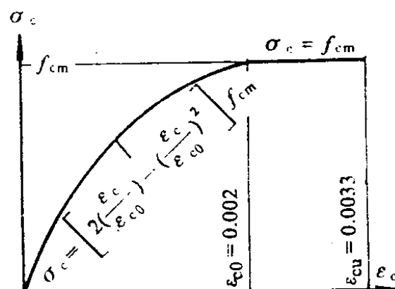
图 2-2 混凝土非均匀受压 应力-应变关系
