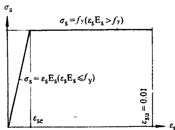
图 2-3 钢筋应力-应变关系
