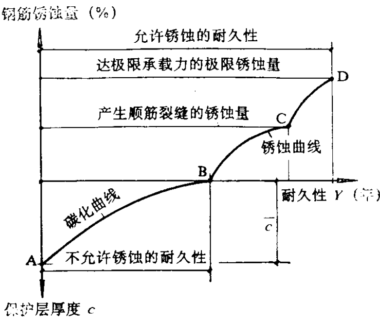
图 1-3 混凝土结构使用寿命
