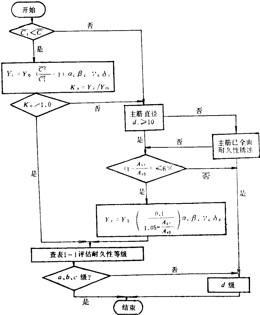
图 1-2 混凝土结构耐久性评估框图
