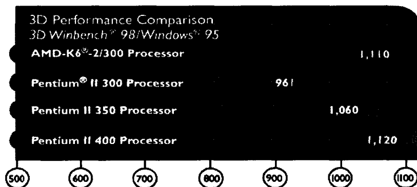
图 0-2：在安装了 Windows 98 之后，K6-2 的 3Dnow! 新指令和 DirectX 6.0 配合，3D 表现上的速度竟然和 Pentium II 400MHz 不相上下，我们在第 3 章会有更详细的介绍。
