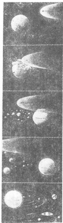
图2 布封假说太阳系形成过程图
