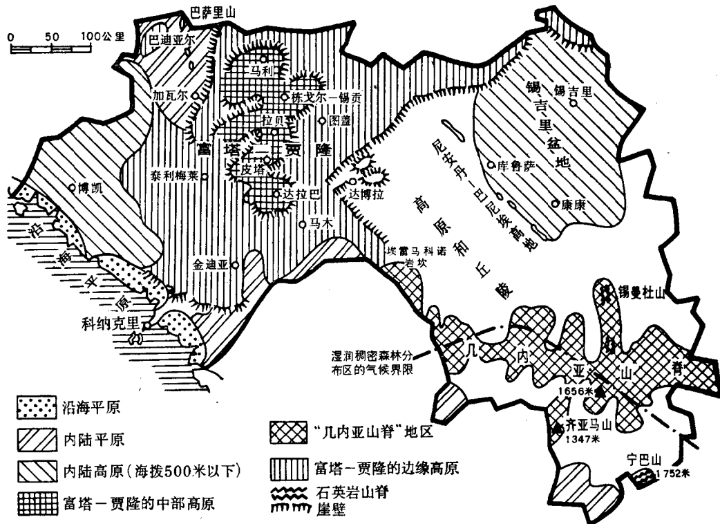
图3 几内亚地貌类型图
