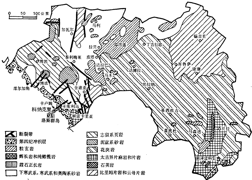
图2 几内亚地质略图
