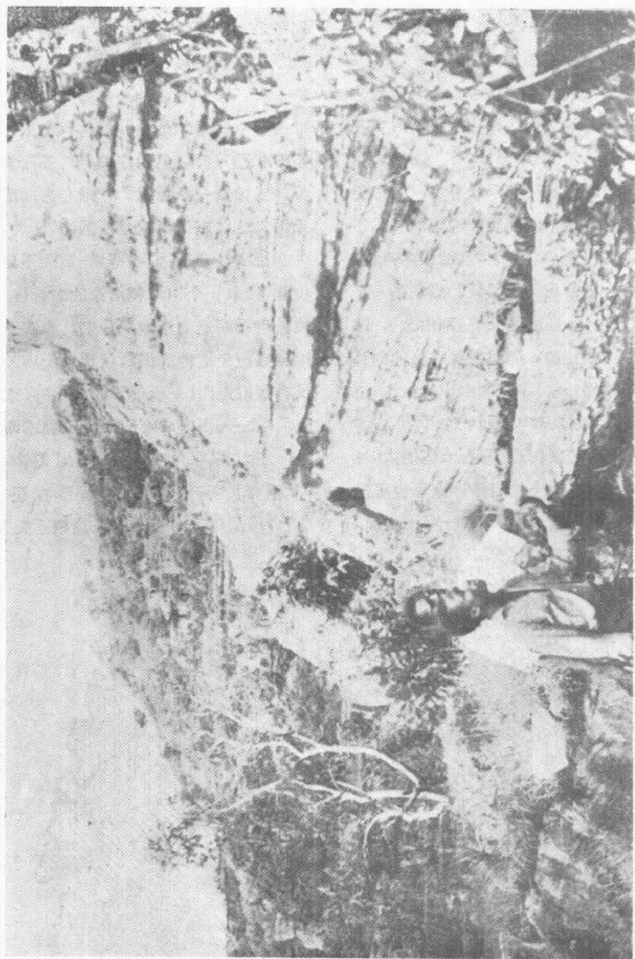
照片 1 富塔-贾隆的砂岩。金迪亚附近甘甘山的山嘴。这是水平产状的薄层砂岩,有些层次是互相穿插的。
