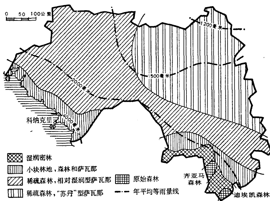
图4 几内亚的植被带和降雨带图
