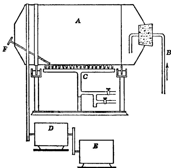
第 1 图 制备无水氢氧化锂的仪器
