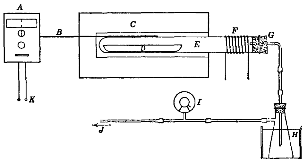
第 2 图 制备氧化锂的仪器
