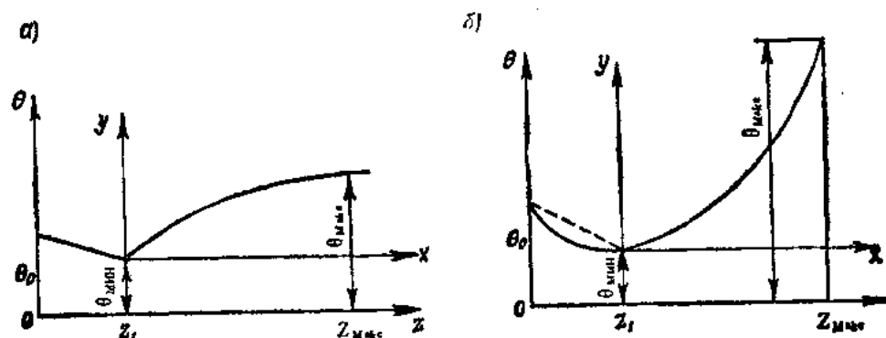
图 2—4 熟地型 (a) 和半螺旋型 (b) 犁体工作面的 \theta = f(z)
