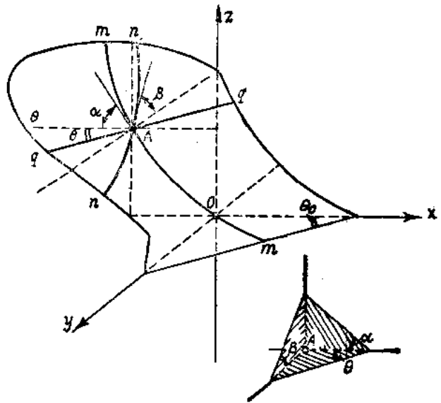
图 2—1 犁体工作面和发展的三面楔
