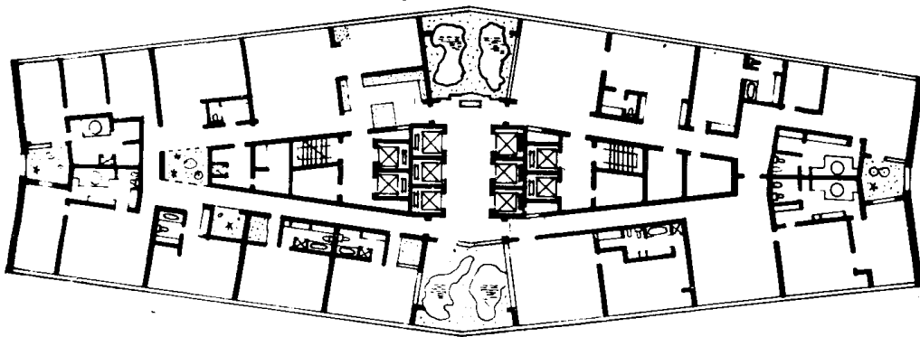
二十八层平面
