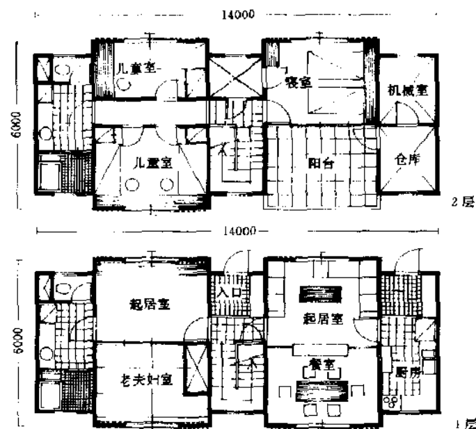
图 1-15 上下卫生空间对正式布局
