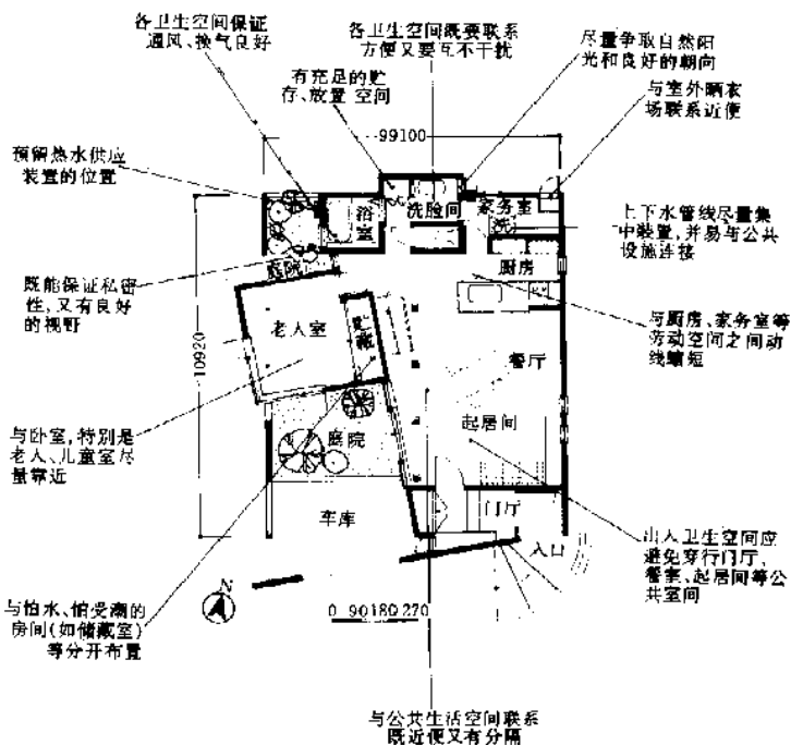
图 1-4 布置卫生空间时应考虑的各种因素
