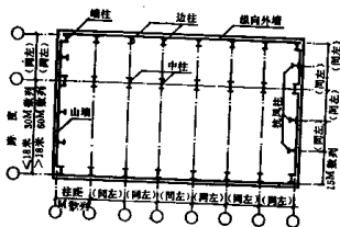
图 13-1 跨度和柱距示意图
