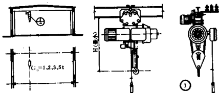
图 12-7 单轨悬挂吊车
