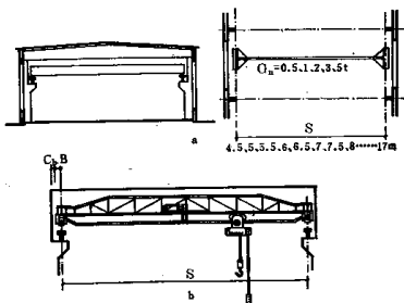
图 12-9 吊车梁支承电动单梁吊车 (DDQ型)
