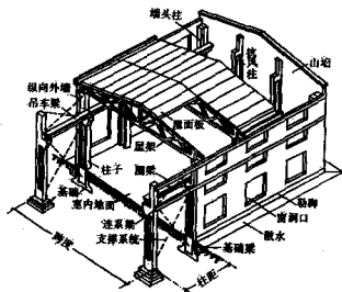
图 12-5 单层厂房的构件组成 (注:未表示屋盖结构支撑系统)
