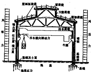
图 12-4 单层厂房结构主要荷载示意
