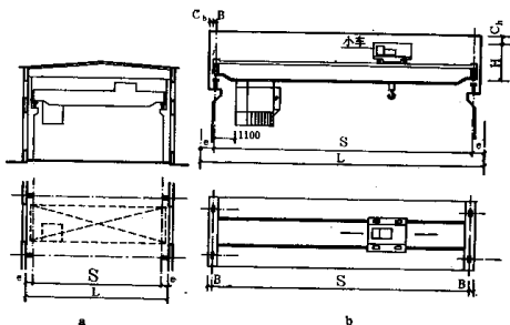
图 12-10 电动桥式吊车 a—平、剖面示意；b—吊车安装尺寸
