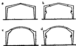
图 12-6 装配式钢筋混凝土门式刚架结构 a—人字形刚架；b—带吊车人字形刚架；c—弧形拱刚架； d—带吊车弧形刚架
