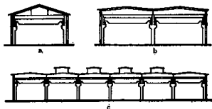
图 12-1 单层厂房
