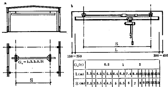
图 12-8 悬挂式电动单梁吊车 (DDXQ型)
