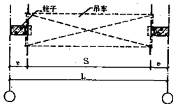
图 13-6 吊车跨度与厂房跨度的关系
