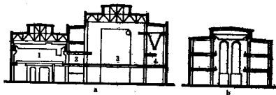
图 12-3 层次混合的厂房
