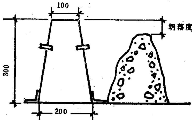
图1-1 混凝土拌合物坍落度试验
