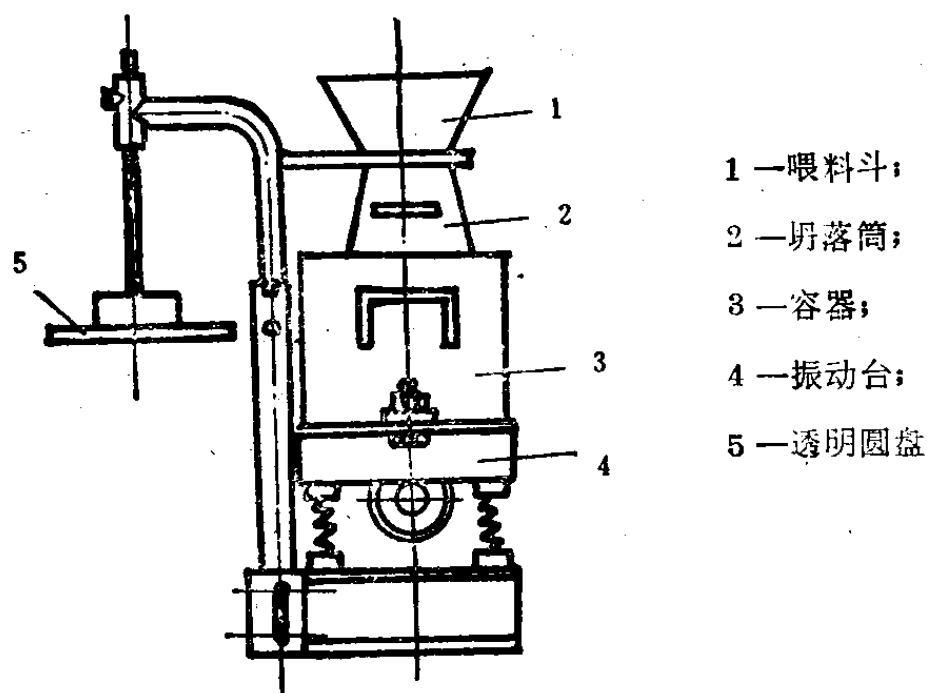
图1-2 维勃稠度仪
