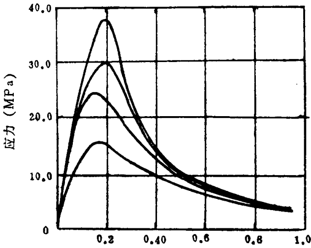
图1-3 混凝土应力—应变全曲线
