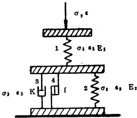
图1-5 混凝土流变性质的复合模型
