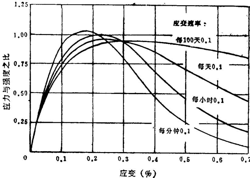
图1-4 应变速率(或加荷速度)对混凝土应力—应变曲线的影响
