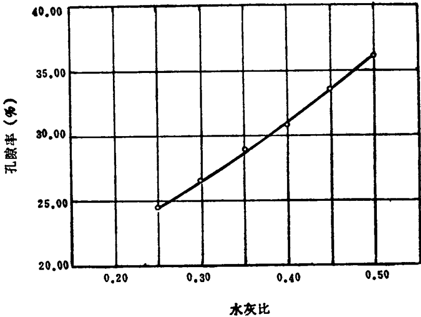
图1-2 水泥石的水灰比与孔隙率的关系
