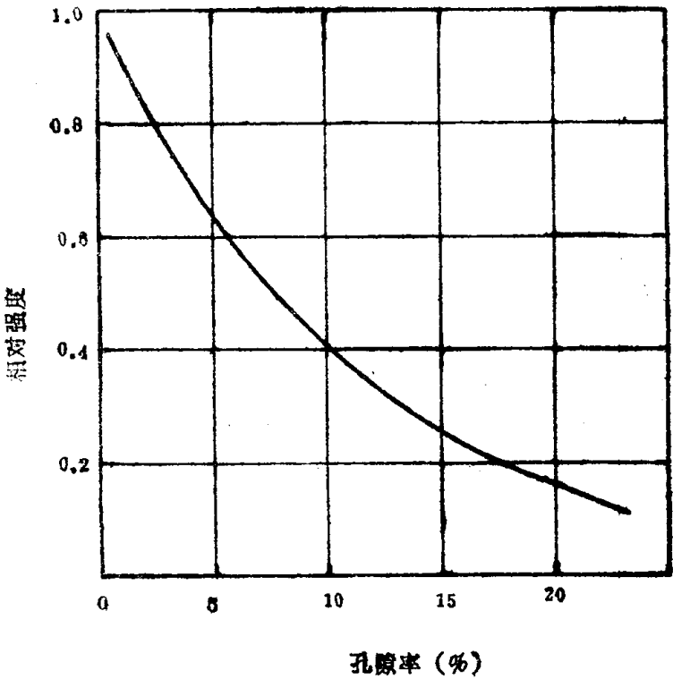
图 1-1 混凝土强度与孔隙率之间的关系
