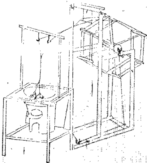
陈启沅设计的缫丝小机
