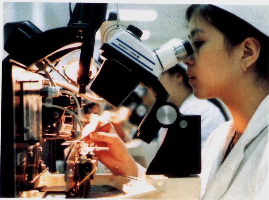
厦门华联电子公司集成电路键合工序
