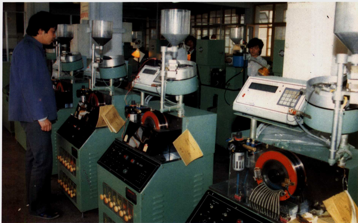
福州无线电元件厂碳膜电阻器生产线
