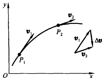
图 1-4 速度的增量
