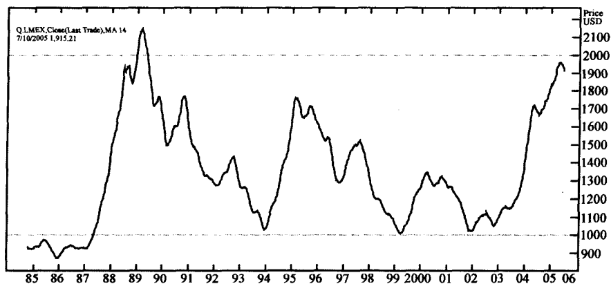
图1-1 伦敦金属指数在2003年突破下降趋势之后强劲上扬
