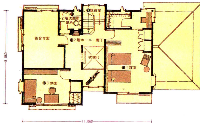
〔2階平面図 S=1/200〕
