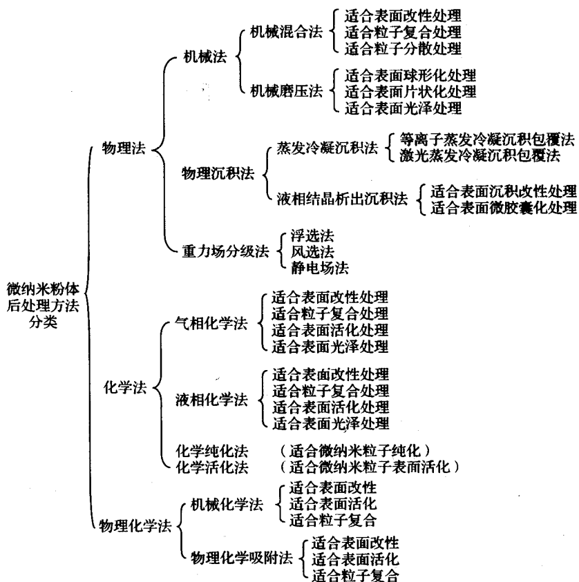
图 1-1 微纳米粉体的后处理方法分类。
