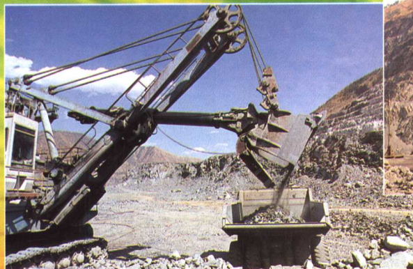
电铲铲装作业
