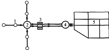
图 1-2 地下水源给水系统
