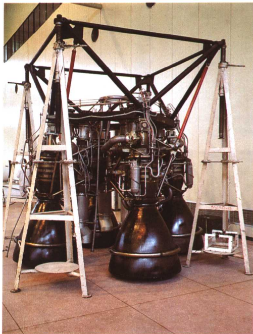
图 49 “长二捆”火箭发动机
