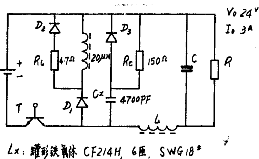
图三 电路实例
