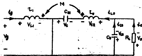
(b) T_{on} 期间等效电路
