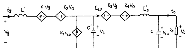
图4 等效的平均电路模型
