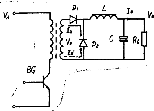
图一 单端开关电源电路
