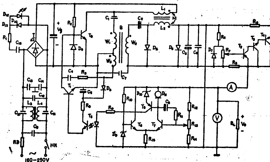
图 1 自激式C'UK-3型稳压电源电路图
