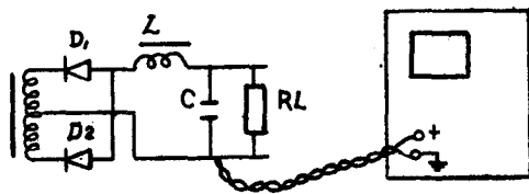
图2. 芯线和地线接触同一点
