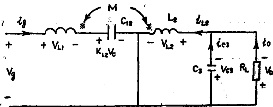
(a) T_{off} 期间等效电路
