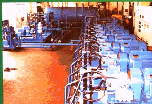
梅山冶金公司步进梁式加热炉液压站
