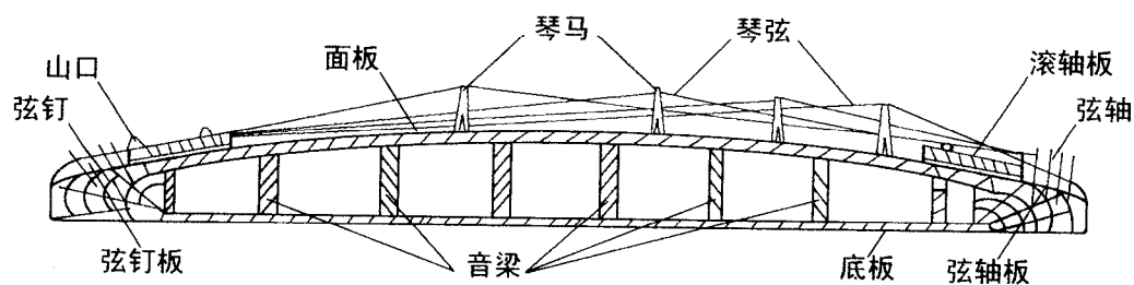
扬琴剖面图
