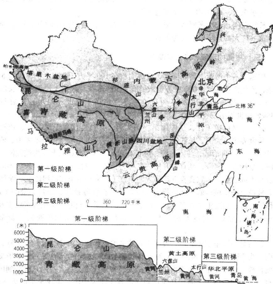
图 1.3 中国山脉分布示意图
