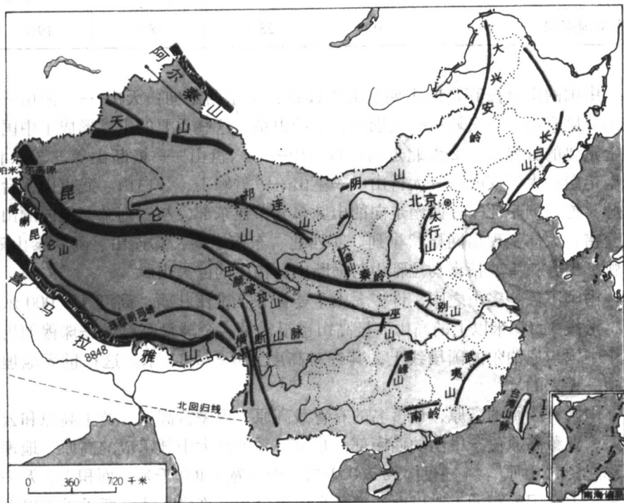
图 1.2 中国地形梯级分布示意图
