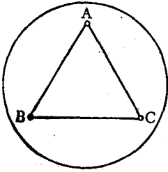
图1-2 汤姆逊的原子模型
