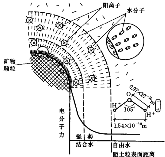
图 1-2 粘粒表面的水
