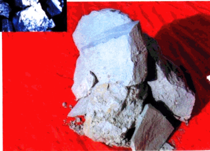
◁ 结晶硅
