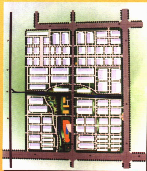
无锡市新区旺庄配套区(二期)规划总平面图
