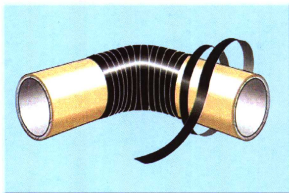
管道防腐材料：热缩缠张带
