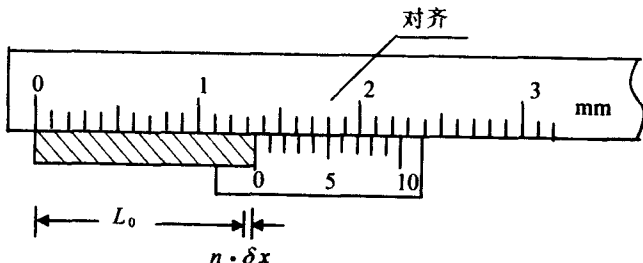
图 1-3 长度测量
