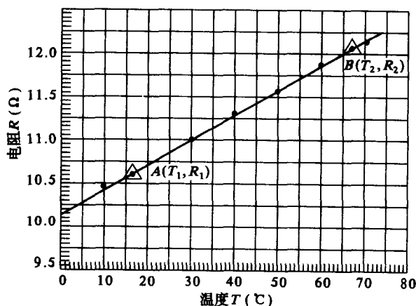
图 2 铜丝的电阻与温度的关系曲线
