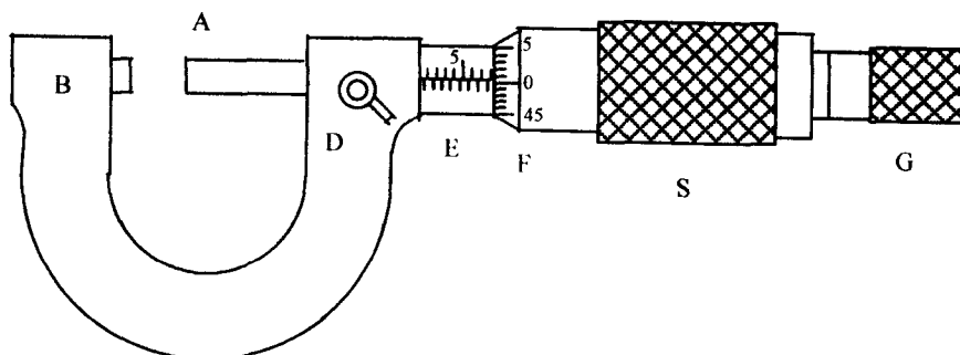
图 1-4 螺旋测微计
