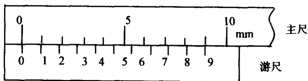
图 1-2 主尺与游标
