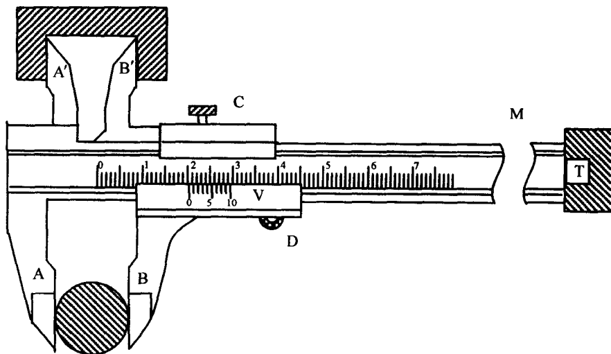
图 1-1 游标卡尺
