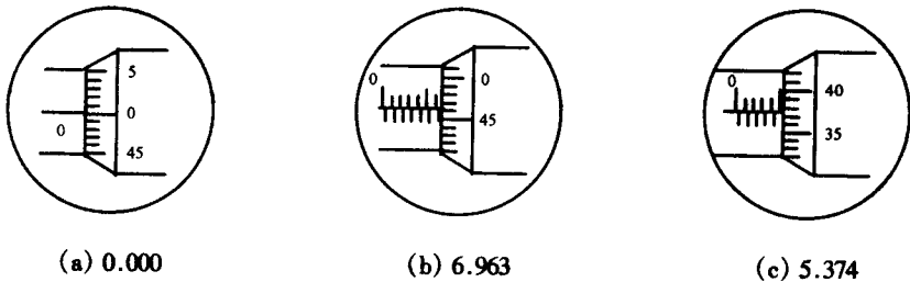
图 1-5 螺旋测微计的读数
