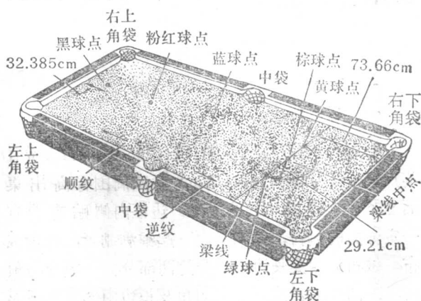
图 1 球桌平面图
