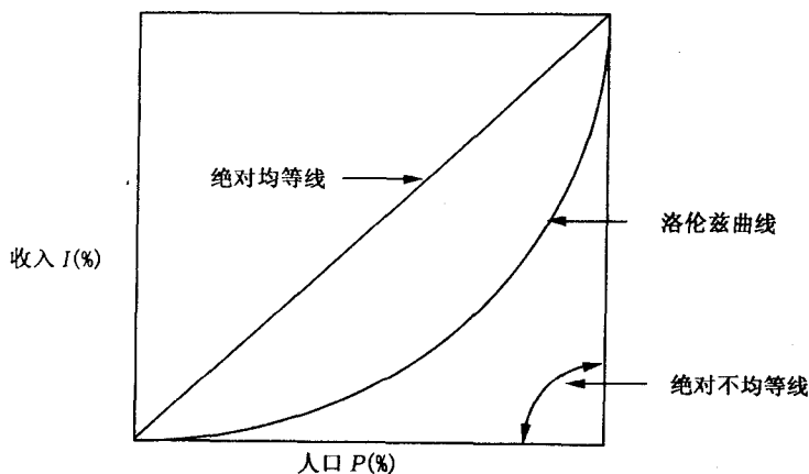
图1-1 洛伦兹曲线
