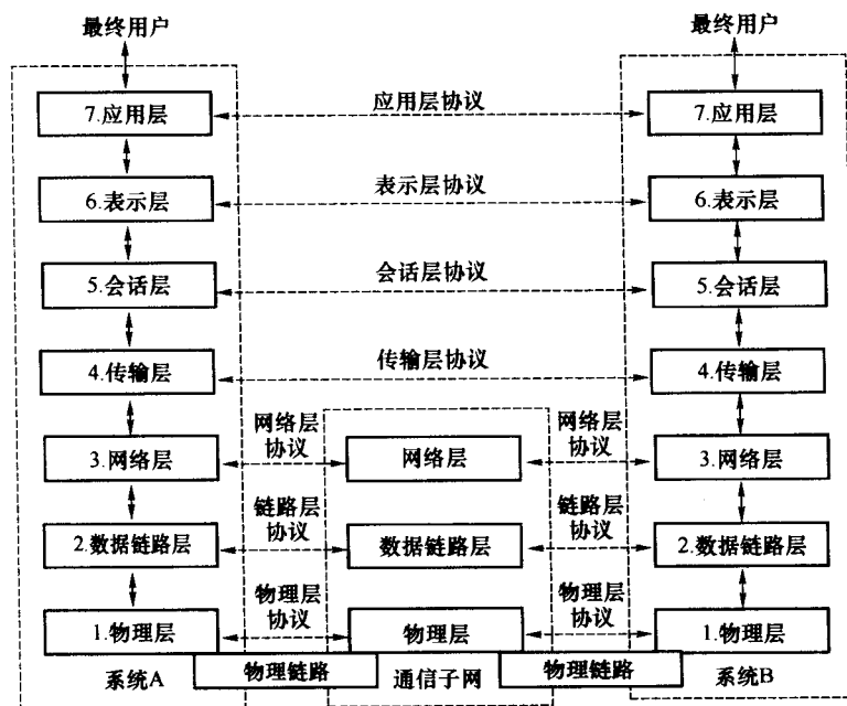
图 1.1.3 系统 A、B 经过子网的通信
