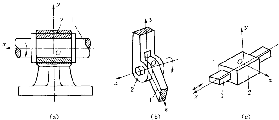
图 2-3 平面低副
