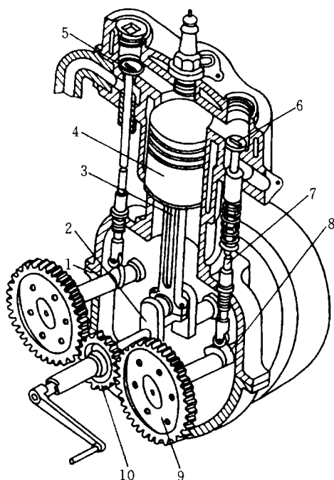
图 1-1 单缸内燃机
