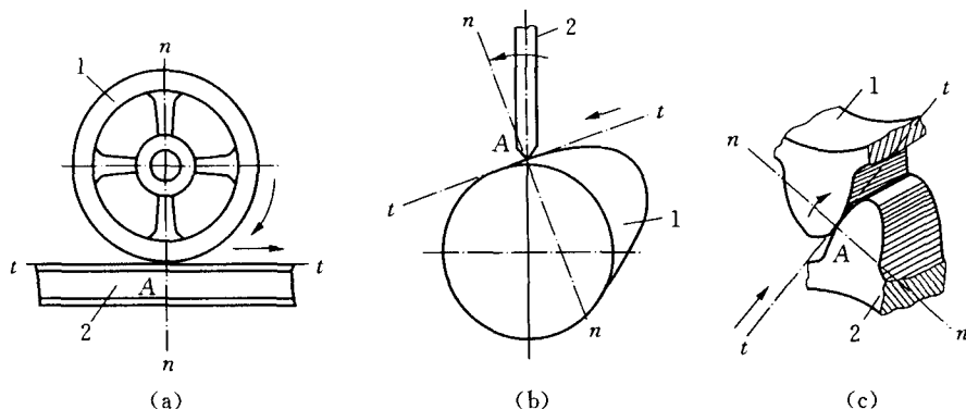
图 2-4 平面高副
