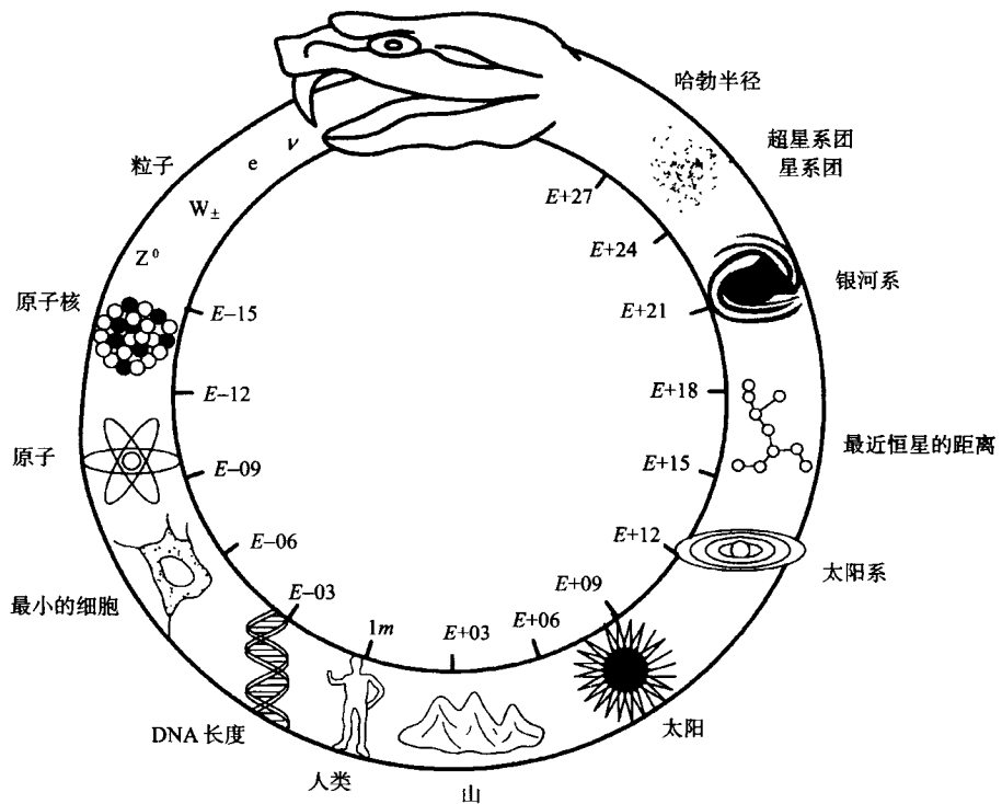
图 1.1 蛇吞尾图,形象地表示了物质空间尺度的层次和宏观系统、微观系统的联系
