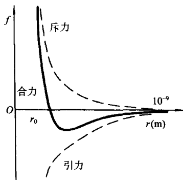
图 1.2 分子间的力与分子间距的关系
