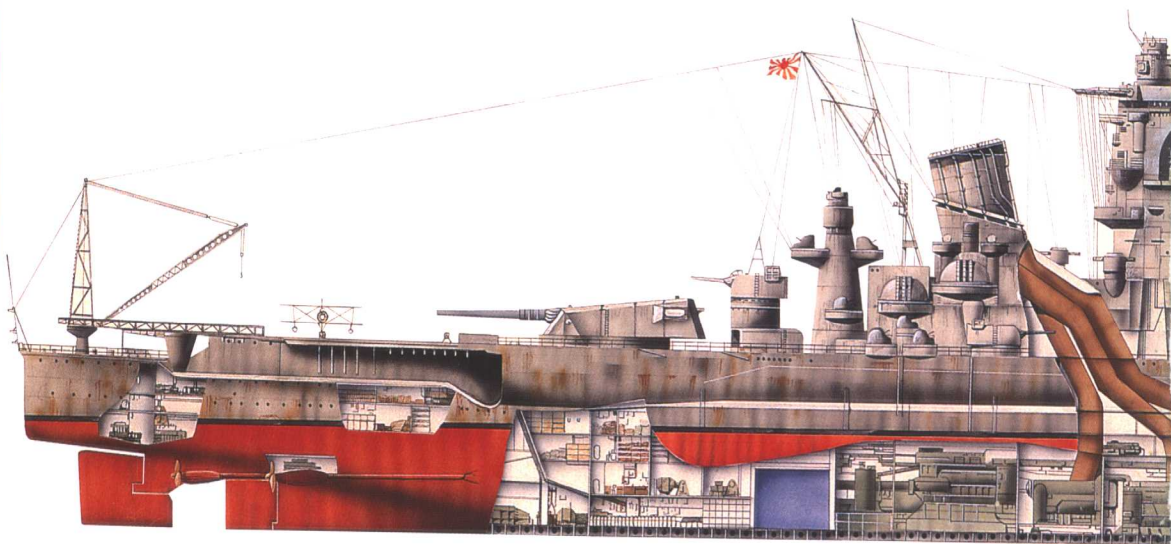
日本“大和”号战列舰
