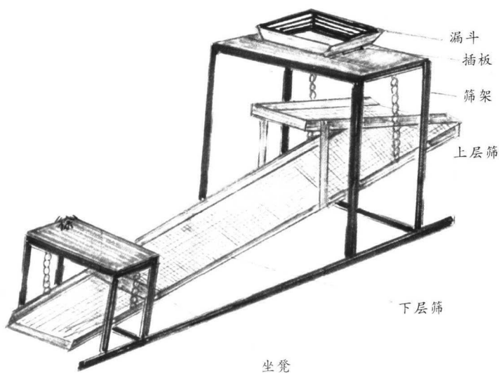
“脚蹬双层流筛”示意图
