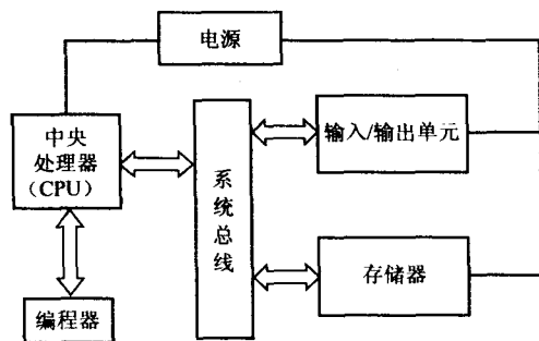
图 1-1 整体式结构
