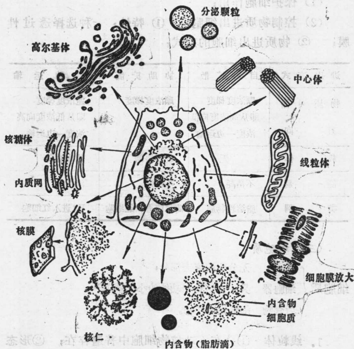
图1-2 真核细胞示意图
