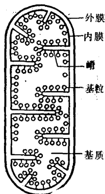
图1-3 线粒体结构
